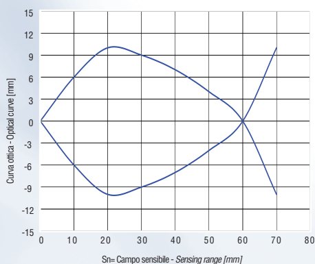
Modello con fibra ottica a tasteggio diretto FPO/D FPO/D optic fiber diffuse type
